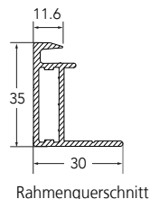
Rahmenquerschnitt
