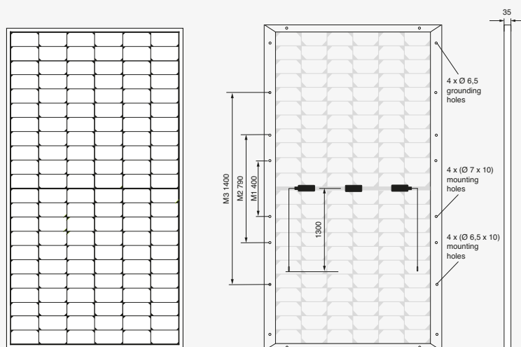
Abb. Prinzipskizze
